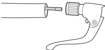
Abbildung 2. Außenhüllenführung aus dem Lenker und in den Bremshebel
