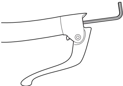
Abbildung 3. Festziehen der Keilschraube an der Hebelklemme
