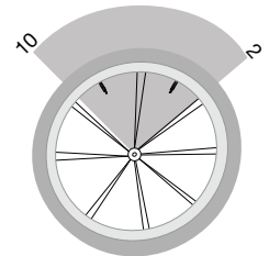
Ilustración 4. Al inflar la rueda, mantenga el vástago de la válvula entre la posición de las 10 y las 2 para que no entre en contacto con SealSafe.
